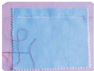
Сметочный шов прямых стежков
