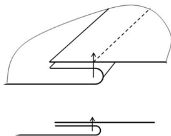
Стачной шов в затяжку
